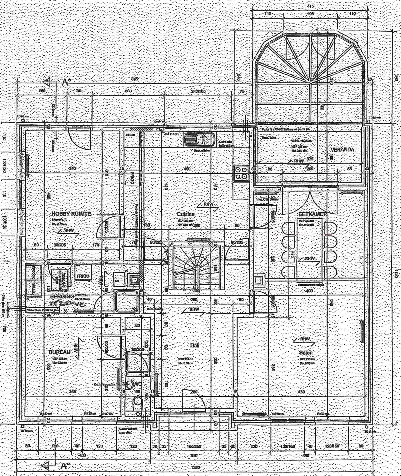
PLAN GELIJKVLOERS VAN NIEKERK
